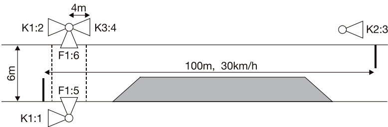
Plan de temporisation de signalisation sans demande piéton :
